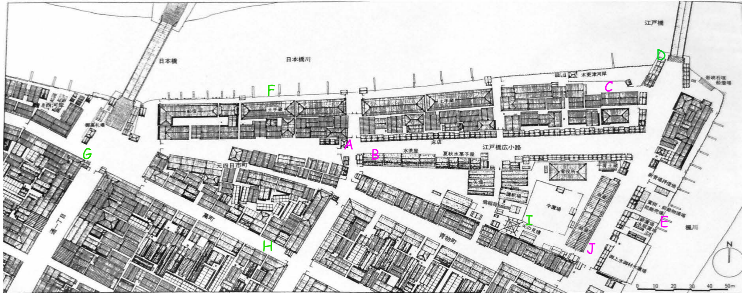
图-9-2 江戸橋広小路復原图（模型全体屋根伏図）
